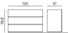
Elemento 3 cassetto P=51 H=78,8
